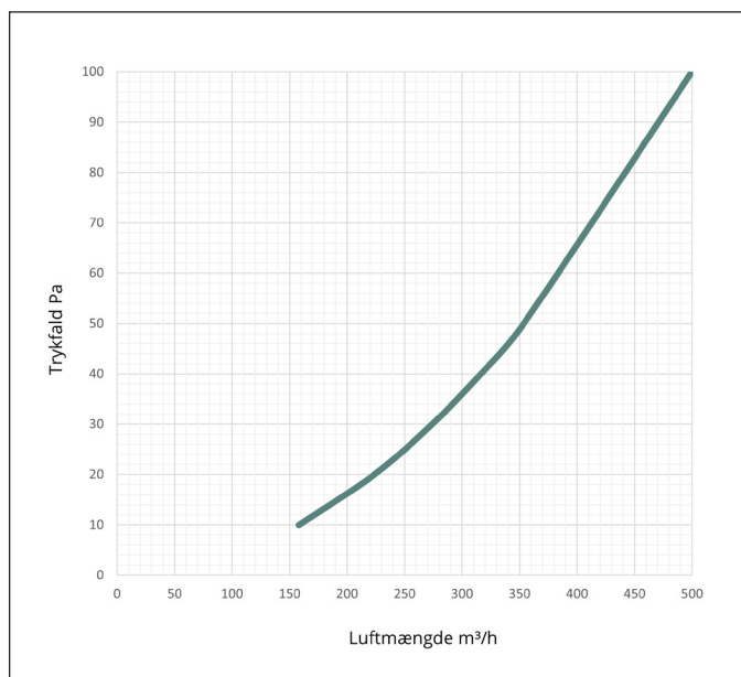
Kapacitetskurve K-faktor 50
