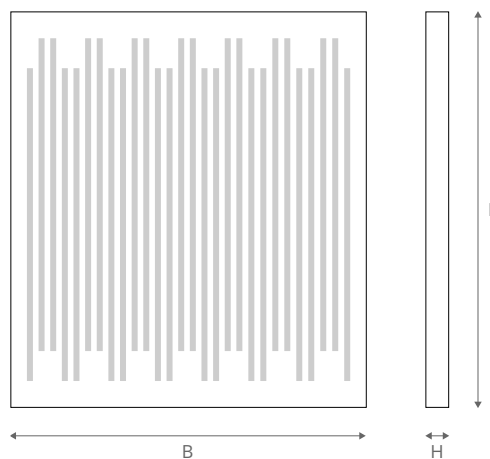
Plantegning
